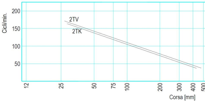
Diagramma cicli/minuto
